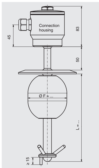
带焊接封盖
