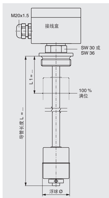
螺纹连接
